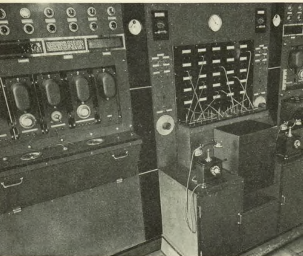
PANEEL VAN HET MODULATIEBORD (GEINSTALLEERD TE BRUSSEL)
