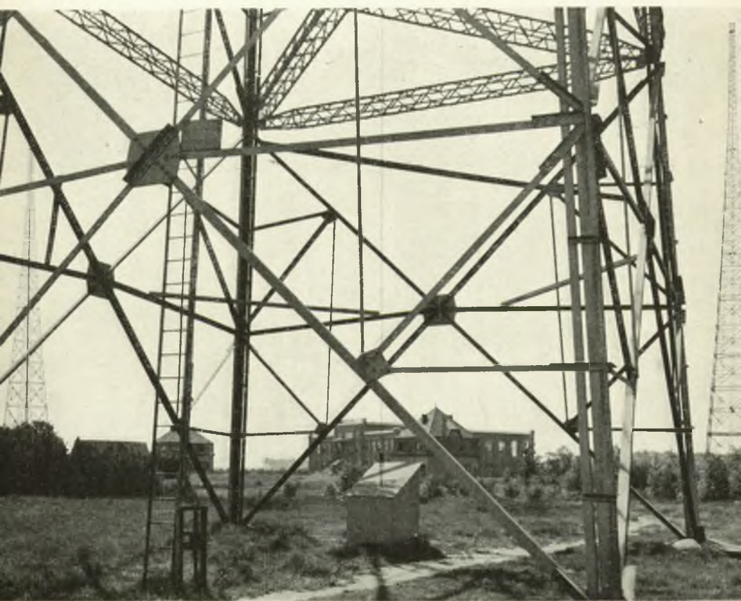
ALGEMEEN GEZICHT OP DE UITZENDINGSSTATIONS TE VELTEM.
