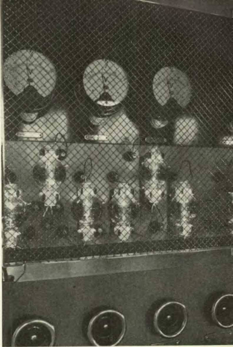
DETAIL VAN EEN PANEEL VAN EEN DER ZENDERS.
